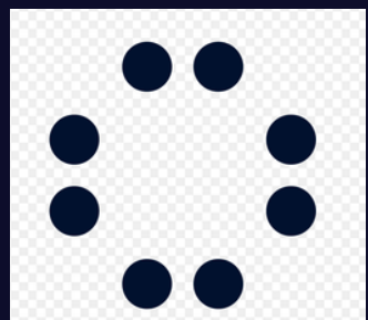
Retell AI
